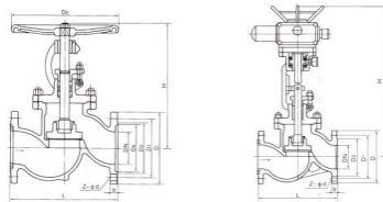
主要外形尺寸及连接尺寸(mm)
